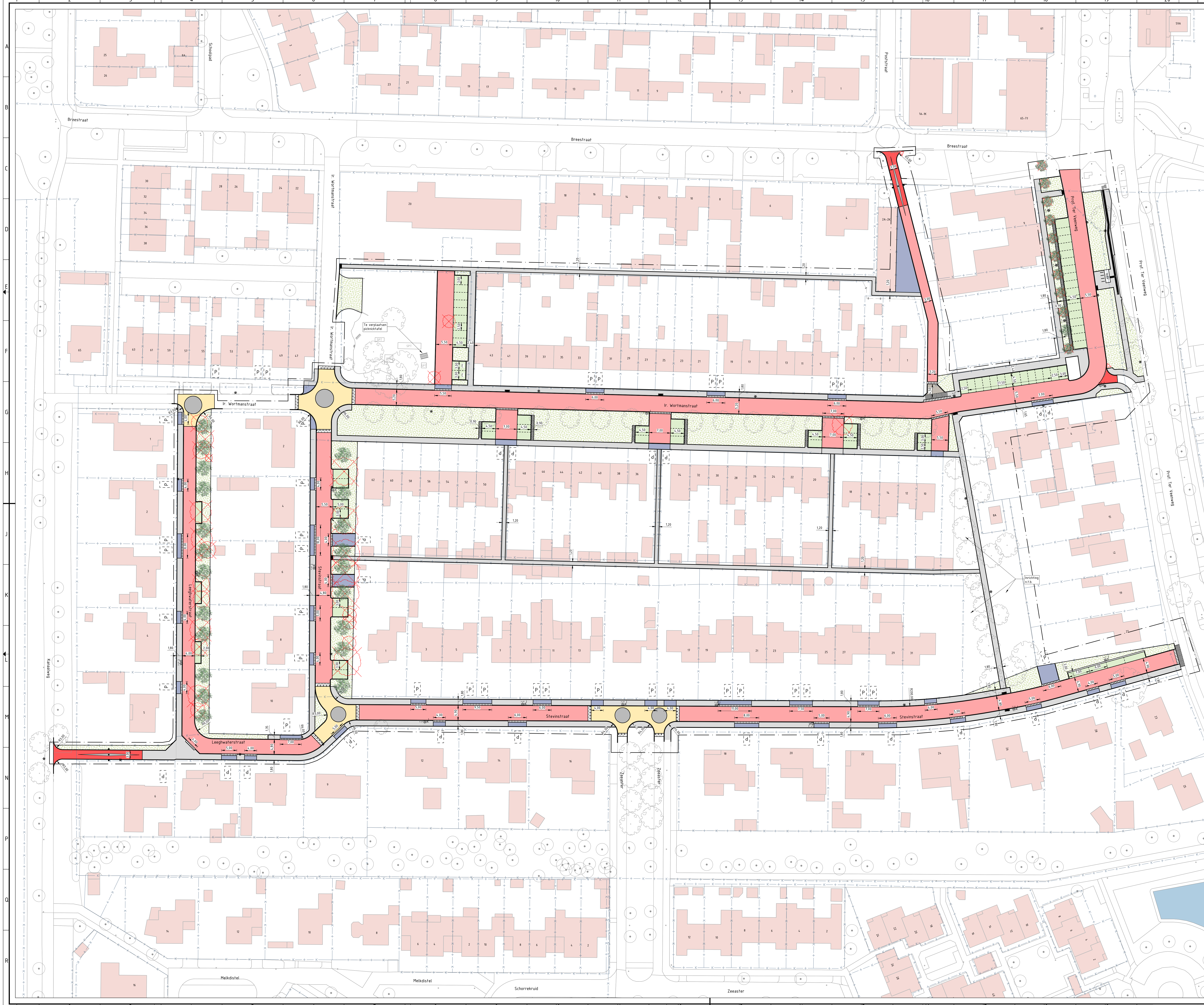
OVERZICHTSTEKENING
