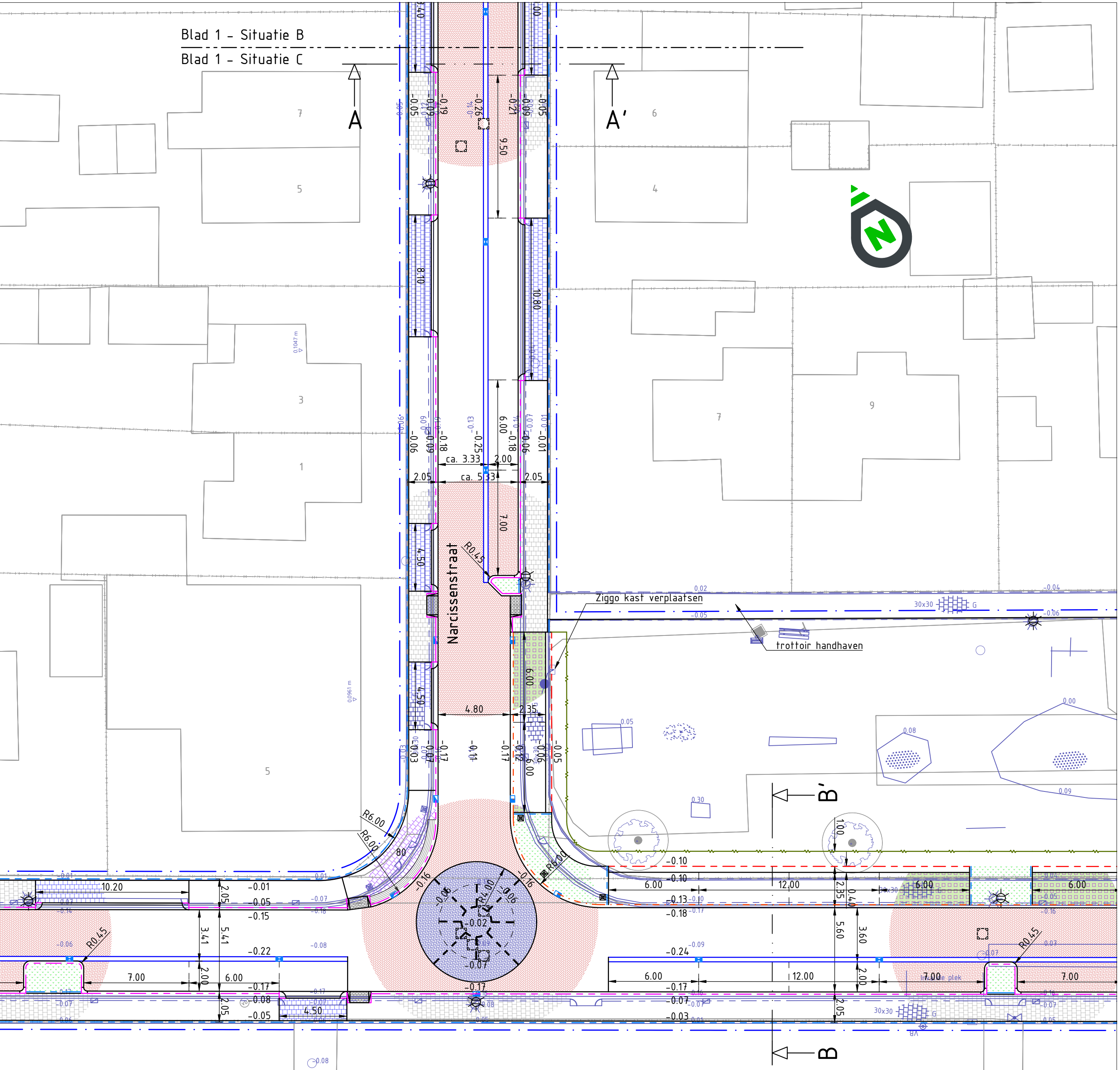
Situatie C SCHAAL 1:200
