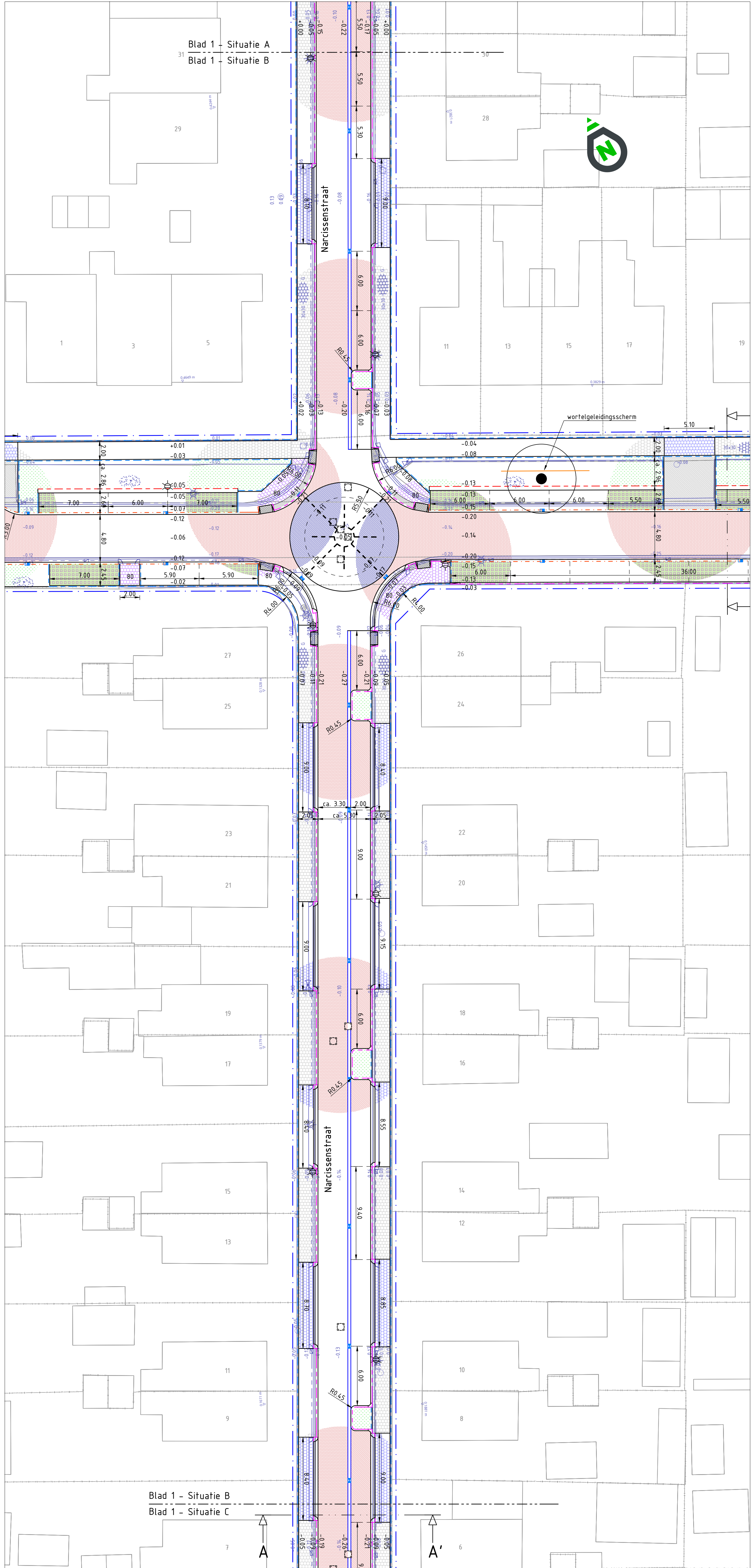
Situatie B SCHAAL 1:200
