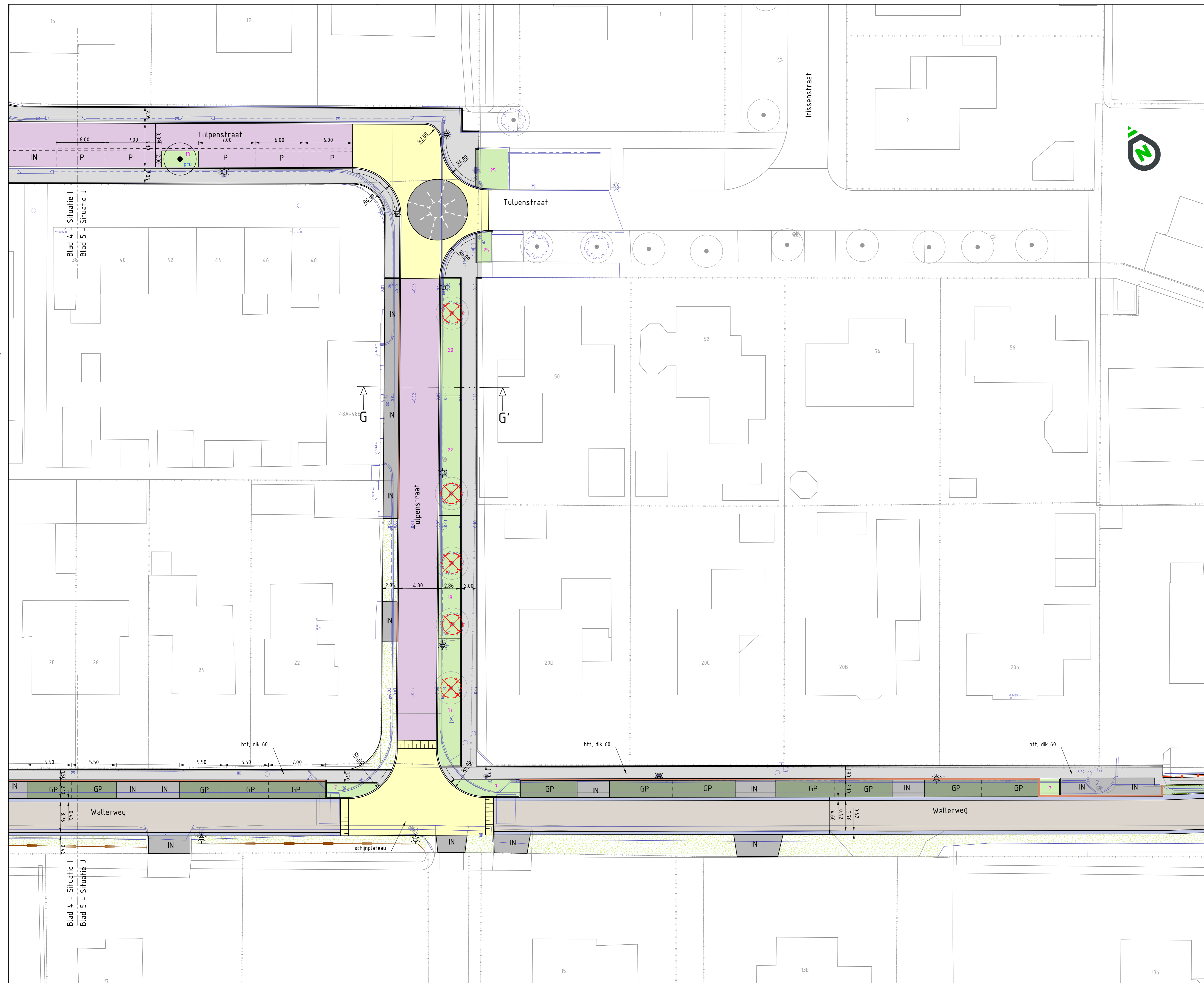
Situatie J SCHAAL 1:200
