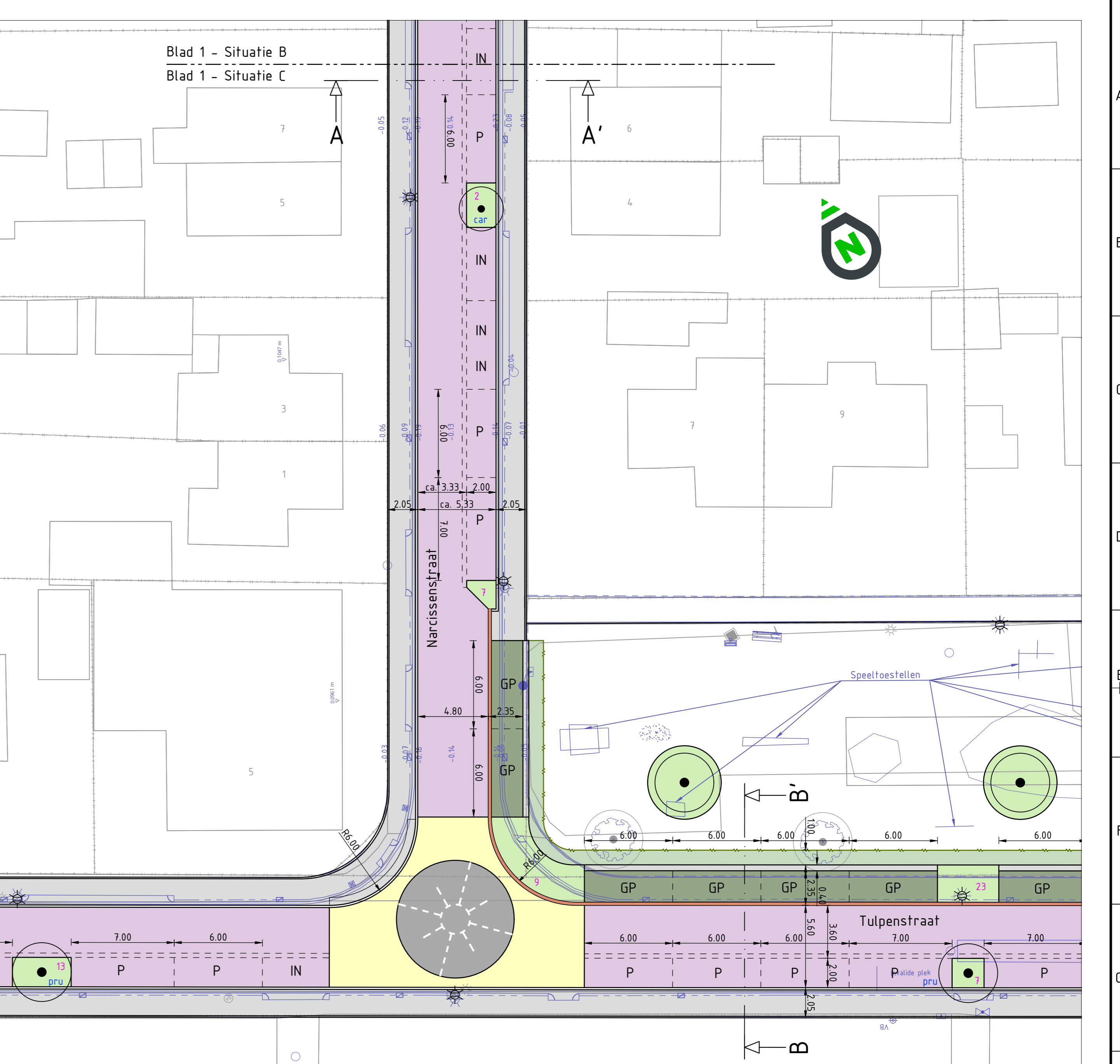
Situatie C SCHAAL 1:200
