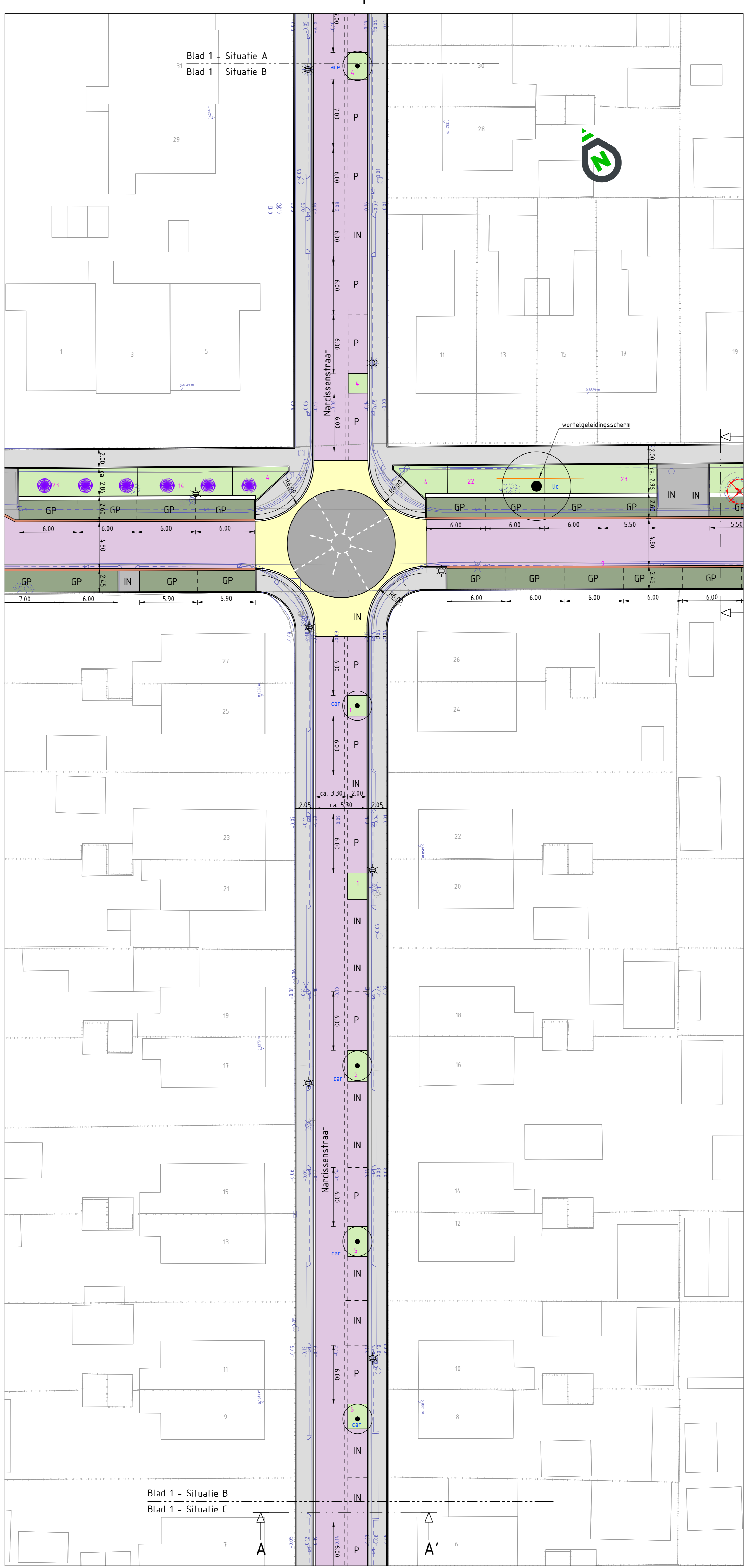
Situatie B SCHAAL 1:200
