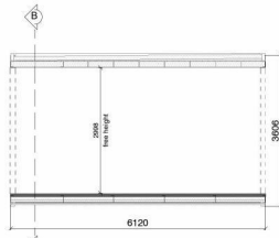
Section A-A schaal 1:50
