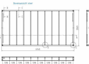
Bovenaanzicht vier
