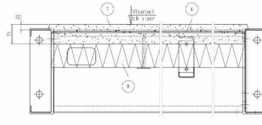
SAFEBEELING VOORCONSTRUCTIE SCHAL 15
