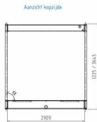
Aanzicht kortzijde
