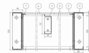
DOORSNEDEN A-A SCHAL 15
