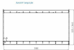
Aanzicht langzijde
