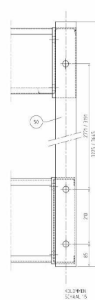
SAFEBEELING VOORCONSTRUCTIE SCHAL 15
