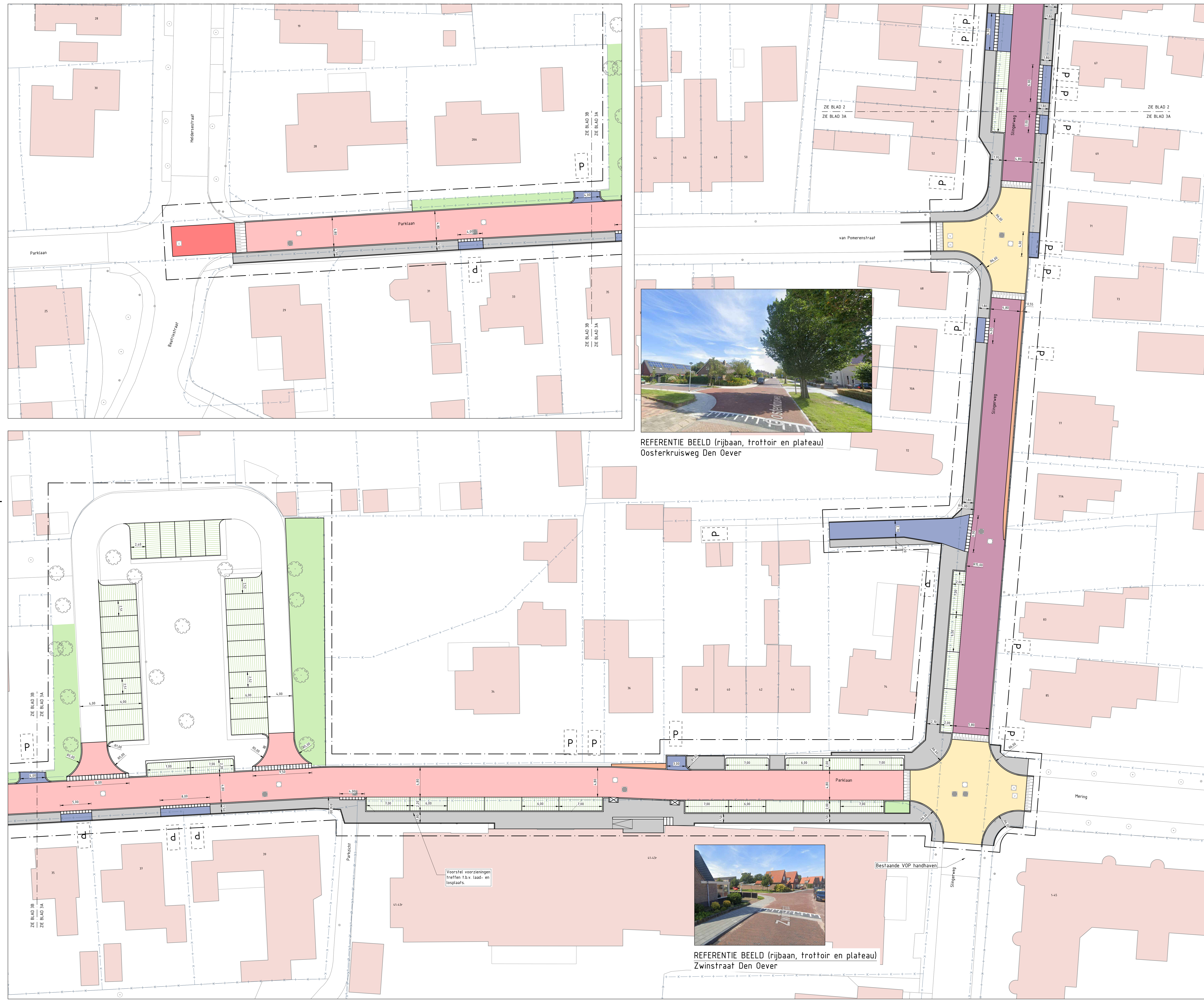
OVERZICHTSTEKENING
