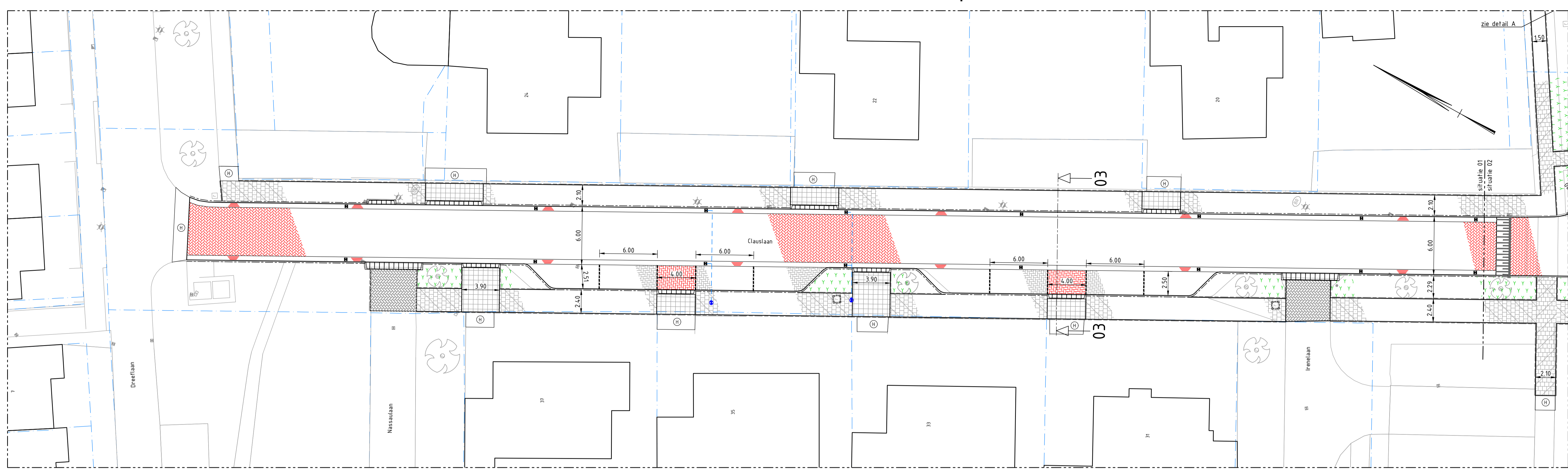
Situatie 01 schaal 1 : 200
